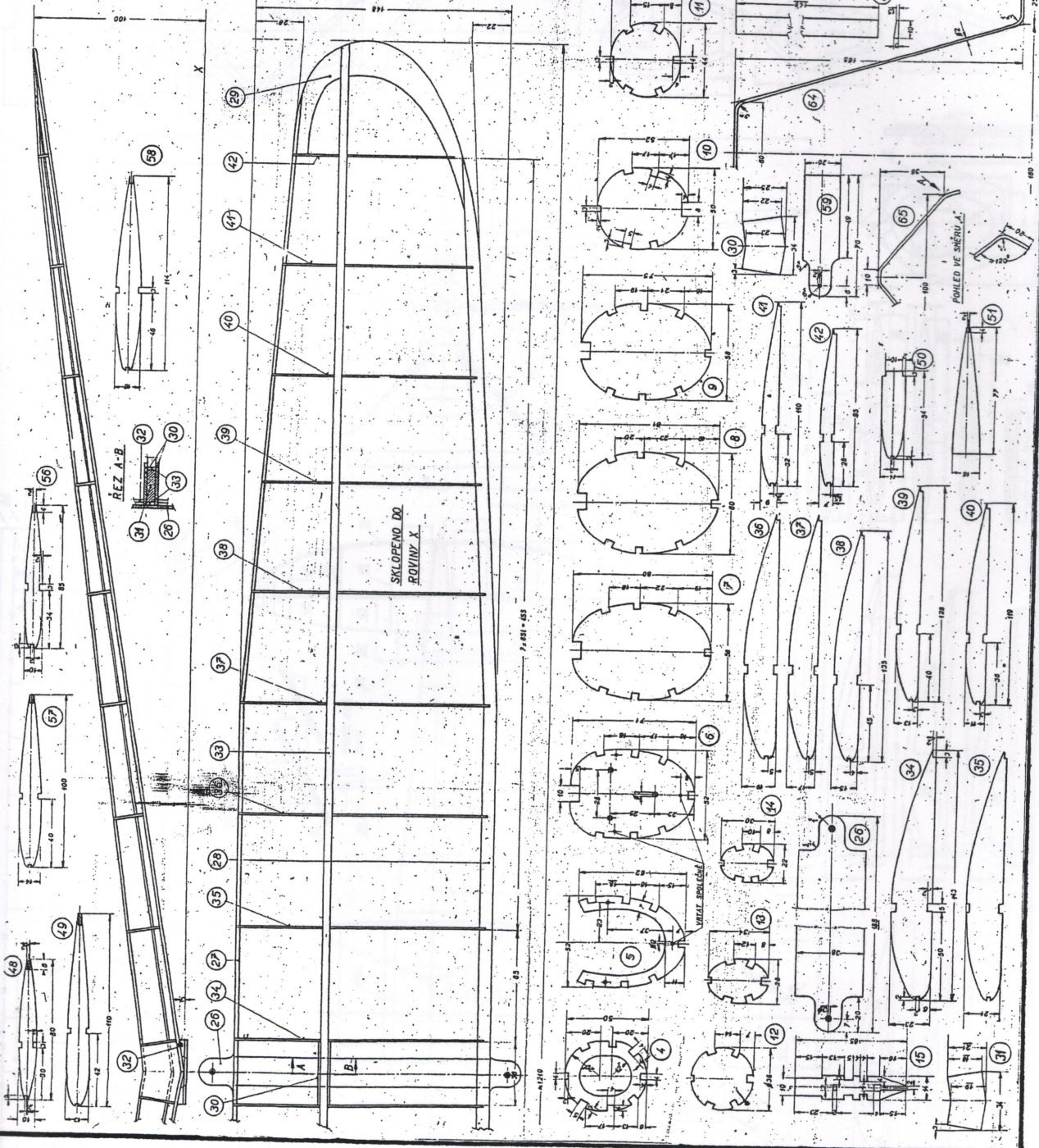
NEKONTOVÉ ROZMĚRY PRŮMĚRY A ŽEBRA POKLÉ MEZUSÍŤEN PŘESNĚJŠÍČÍSKA.
